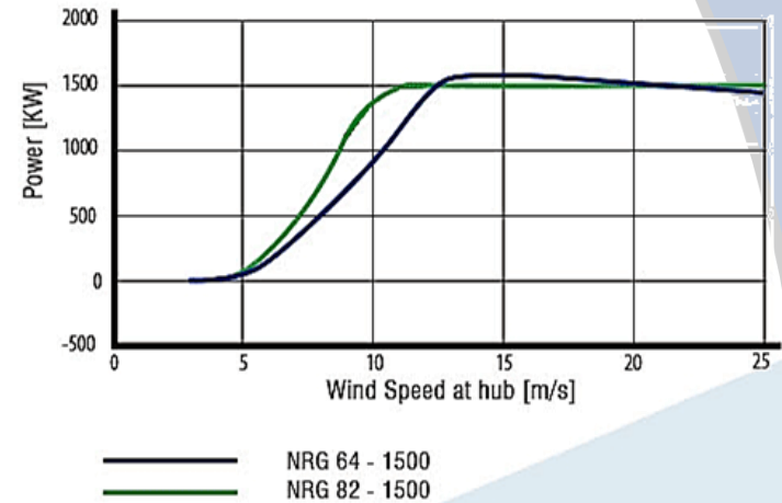
CURVA DE POTENCIA NRG 1500 Clase I (64 - 1500) y Clase II (82 - 1500)
